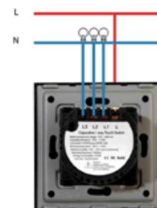
ЕДНОНАСОЧНО ПОВРЗУВАЊЕ
