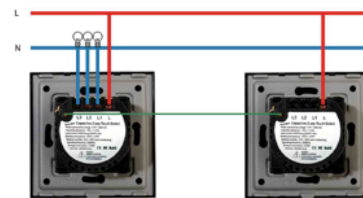
ДВОНАСОЧНО ПОВРЗУВАЊЕ
